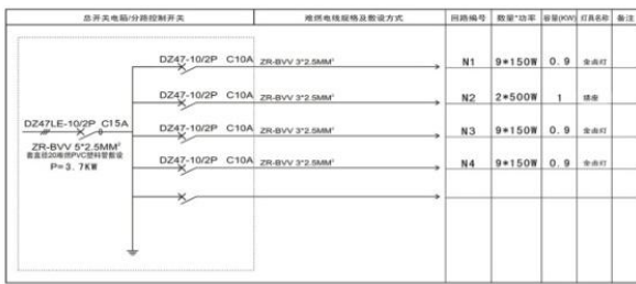
中国婚博会展位配电系统图
