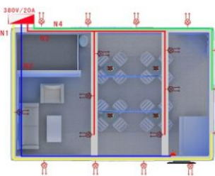
电气平面布置图
